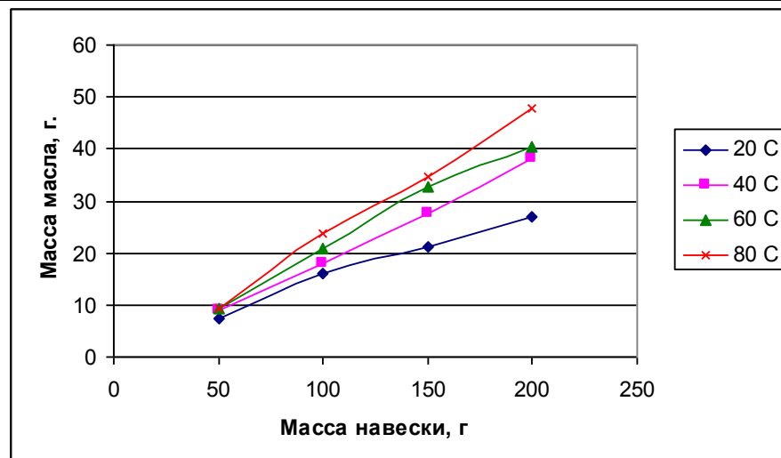
Рисунок 1. Влияние массы навески на массу собранного масла
